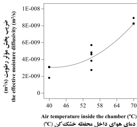
شکل (۵) اثر خطی دمای هوای محفظه خشک کن بر ضریب انتشار مؤثر رطوبت ورقه های قارچ دکمه ای خوراکی
