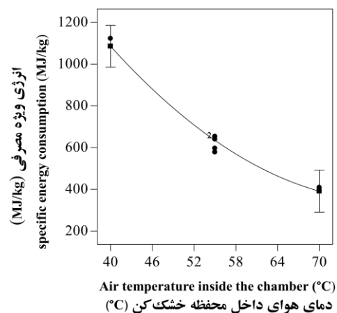
شکل (۶) اثر خطی دمای هوای محفظه خشک‌کن بر انرژی ویژه مصرفی ورقه‌های قارچ دکمه‌ای خوراکی Figure (6) The linear effect of drying room air temperature on specific energy consumption of edible button mushrooms
