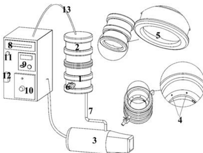
شکل (۱) شماتیک خشک‌کن خلاء- مادون قرمز (۱-۲) محفظه خلاء، ۳- پمپ خلاء، ۴- حسگرهای دما و خلاء، ۵- لامپ مادون قرمز، ۶- ترموستات، ۷- سوپاپ هوای ورودی، ۸- لوله‌های خلاء، ۹- سیستم کنترل فشار، ۱۰- ترموستات، ۱۱- دایمر، ۱۲- چراغ سیگنال، ۱۳- فیوز، ۱۴- کابل برق
