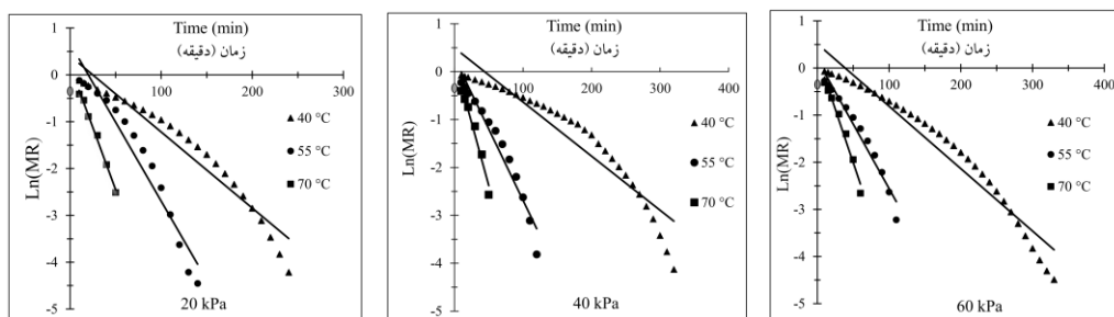
شکل (۴) \text{Ln}(\text{MR}) خشک کردن لایه‌های نازک قارچ دکمه‌ای خوراکی با خشک‌کن خلأی - مادون قرمز در فشار و دماهای مختلف
