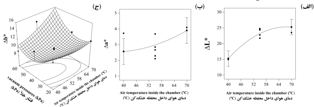
شکل (۸) اثر خطی و متقابل دمای هوای ورودی به خشک‌کن و فشار خلأ بر شاخص‌های رنگی پودر قارچ دکمه‌ای (الف) - \Delta L^* ب- \Delta a^* و ج- \Delta b^*
