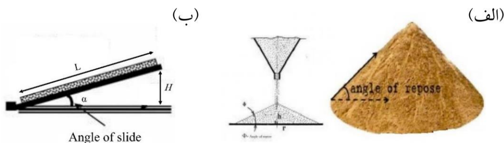
شکل (۲) الف - شماتیک اندازه‌گیری زاویه ریوز، ب - شماتیک اندازه‌گیری زاویه اصطکاک سطحی Figure (2) a- Schematic of the angle of repose b- schematic of slide angle measurement
