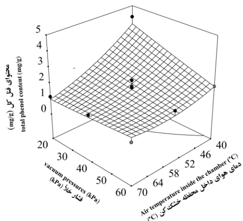
شکل (۷) اثر متقابل دمای هوای داخل محفظه خشک کن و فشار خلأ بر محتوای فنل کل پودر قارچ دکمه ای خوراکی
