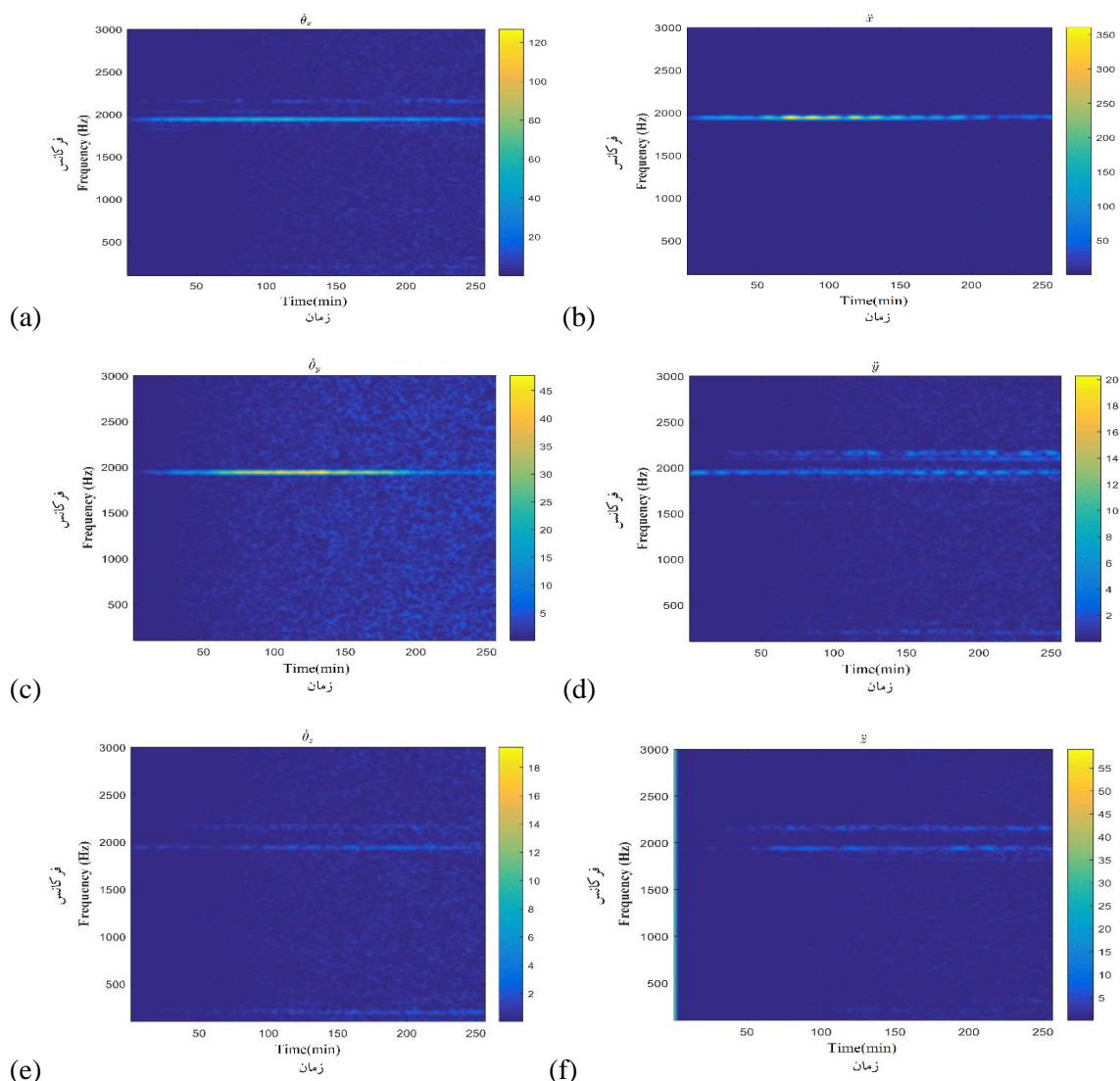
شکل (۴) اسپکتروگرام حاصل از ضرایب کپستروم مل فرکانس. (a)، (c) و (e): به ترتیب سرعت زاویه‌ای در راستای محور X، Y و Z؛ (b)، (d) و (f): شتاب در راستای محور X، Y و Z
