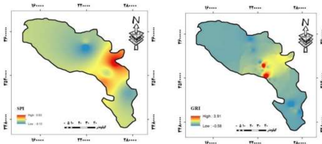
شکل (۲): پهنه‌بندی شاخص SPI و GRI در سال ۲۰۰۶
