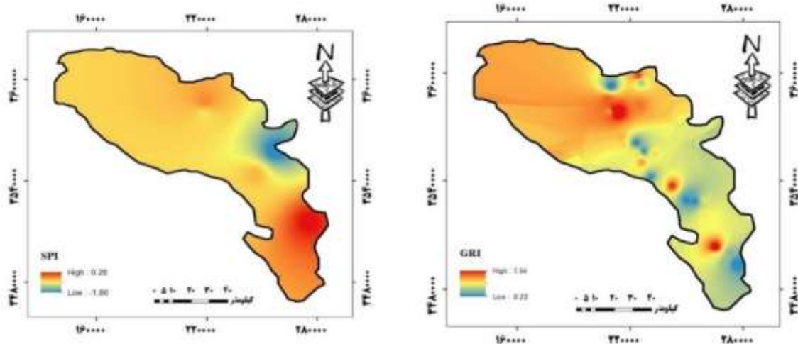
شکل (۴): پهنه‌بندی شاخص SPI و GRI در سال ۲۰۱۴
