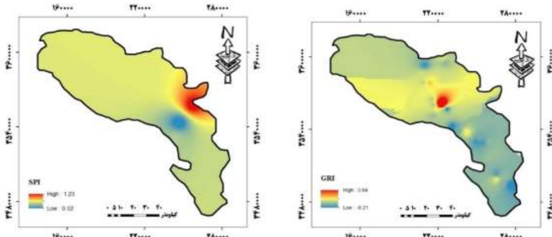
شکل (۳): پهنه‌بندی شاخص SPI و GRI در سال ۲۰۱۰
