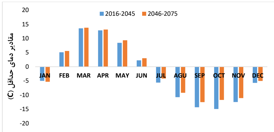
شکل (۵): تغییرات دمای حداقل طی دو بازه زمانی و بر اساس سناریو ۴/۵
