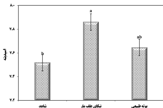
شکل (۱۶): مقایسه میانگین مقدار اسیدیتته خاک در سه واحد اراضی مورد مطالعه
