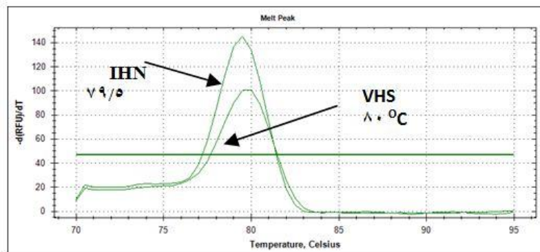
شکل ۳: نتایج منحنی نقطه ذوب آغازگرهای VHS و IHN در نمونه های آزمایشی ماهیان مزارع مختلف با استفاده از کیت Nova SYBR Green
