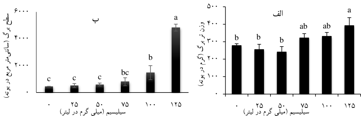
شکل ۲- تغییرات وزن تر برگ (الف) و سطح برگ (ب) در بوته بادرنجبویه به غلظت‌های مختلف سیلیسیم محلول غذایی در
