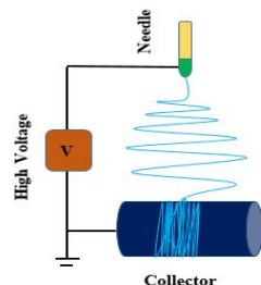
تصویر شماره 1: تصویر شماتیک فرآیند الکترورسی
