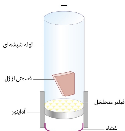
شکل ۲. نمای شماتیک الکتروالوشن پروتئین
