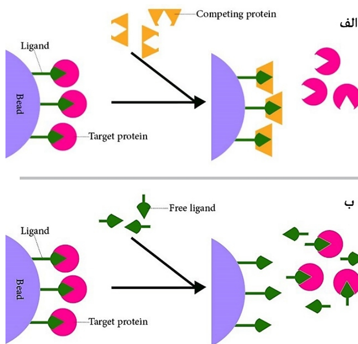
شکل ۱۲. آزادسازی پروتئین‌های هدف به وسیله پروتئین‌های رقیب (الف) و لیگاندهای رقیب (ب)
