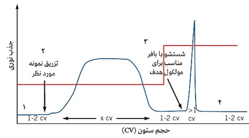
شکل ۱۱. تصویر شماتیک از کروماتوگرافی تمایلی و نمودار حاصل از آن [۱۶]
