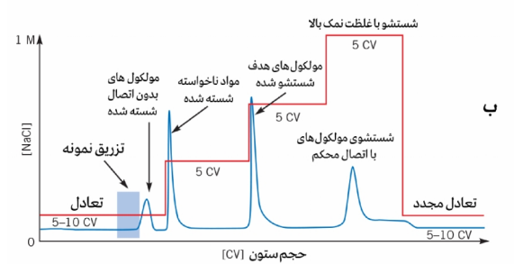
شکل ۹. کروماتوگرافی تعویض یونی [۱۶]
