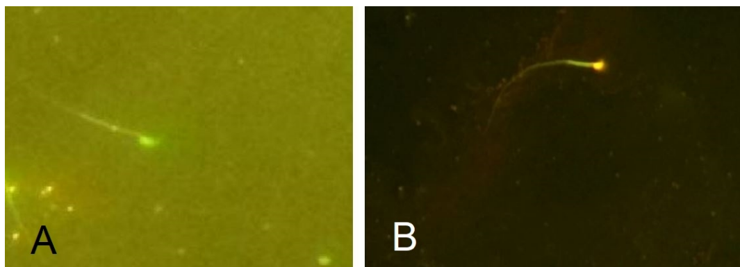
شکل ۲. ارزیابی تمامیت DNA در اسپرمها؛ (A) اسپرمهای با سر سبز رنگ نشان دهنده DNA طبیعی و دست نخورده می باشد؛ (B) اسپرمهای با سر نارنجی نشان دهنده DNA دناتوره شده می باشد. رنگ آمیزی آکریدین اورنج. بزرگنمایی 200X
