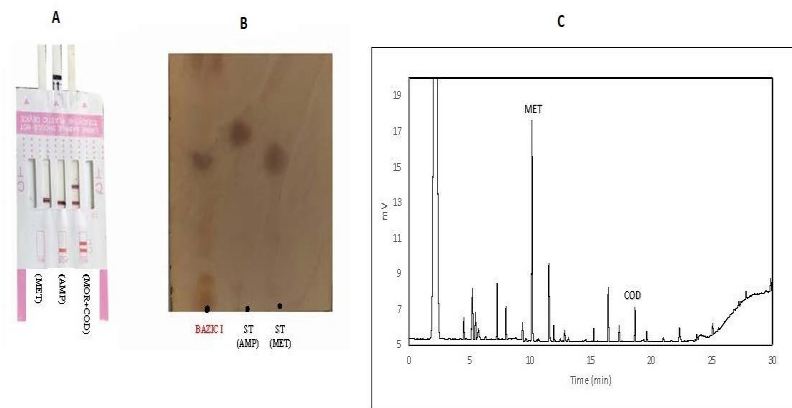
شکل ۲. نتایج مربوط به نمونه حقیقی I قلبایی، A- ICG، B- پلیت TLC، C- کروماتوگرام GC
