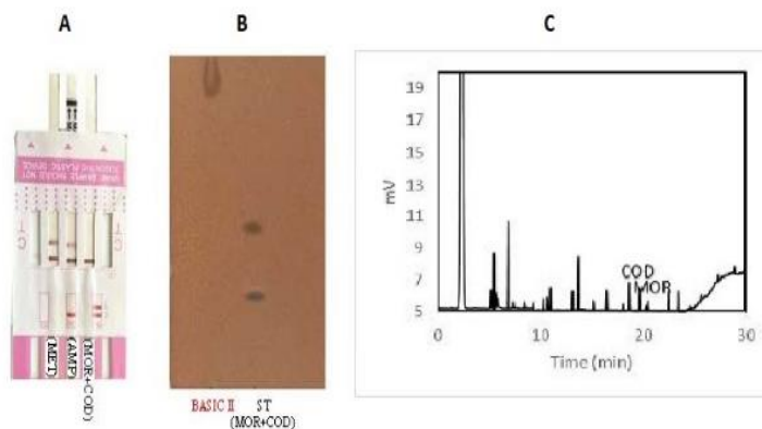
شکل ۳. نتایج مربوط به نمونه حقیقی II قلبایی، A- ICG، B- پلیت TIC، C- نمودار کروماتوگرام GC
