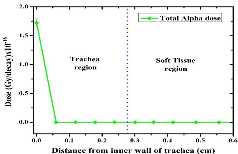
شکل ۳. پروفایل دوز مربوط به مشارکت تمام دخترهسته‌های آلفای زنجیره واپاشی رادون به ازای هر واپاشی
