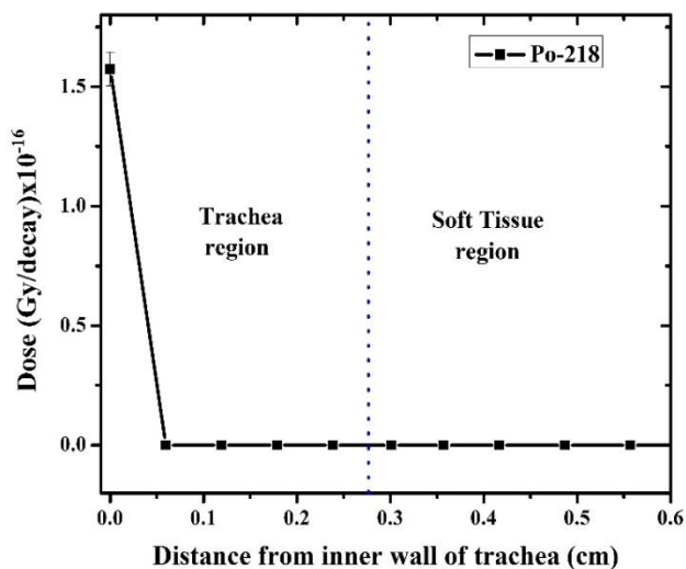
شکل ۲. پروفایل دوز مربوط به دخترهسته‌های آلفای زنجیره واپاشی رادون به ازای هر واپاشی گاز رادون
