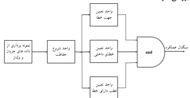
شکل ۲: دیگرام بلوکی حفاظت پیشنهادی.
