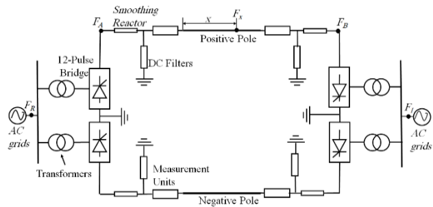
شکل ۱: سیستم دو قطبی [۱].
