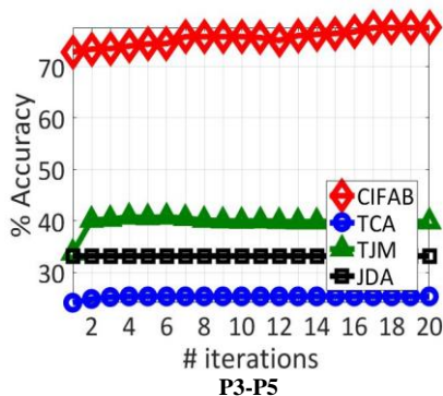
شکل ۴: ارزیابی دقت روش‌های CIFAB و TCA، JDA، TJM، NN در پایگاه داده‌های P3-P5، C-A، U-M در ۲۰ تکرار
