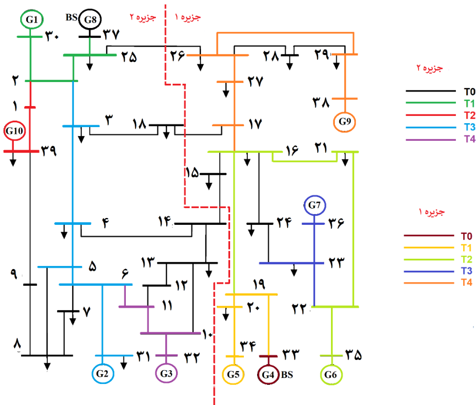
شکل ۵: جزیره‌سازی و فرایند بازگردانی سیستم ۳۹ شینه IEEE (مورد مطالعاتی اول)
