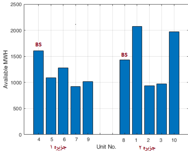
شکل ۴: قابلیت تولید انرژی واحدهای سیستم ۳۹ شینه IEEE در ۱۸۰ دقیقه اول فرایند بازگردانی (مورد مطالعاتی اول)
