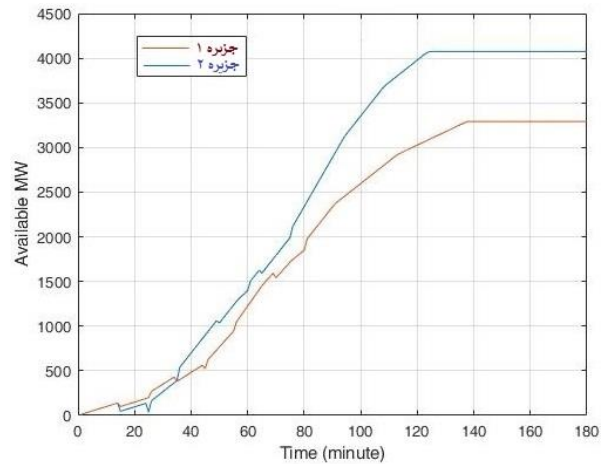
شکل ۳: قابلیت تولید توان در هر یک از جزیره‌ها حین فرایند بازگردانی سیستم ۳۹ شینه IEEE (مورد مطالعاتی اول)
