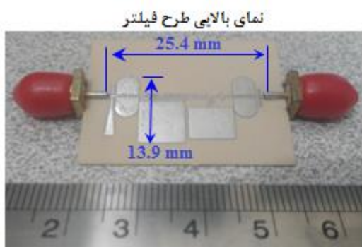
شکل ۱۰: نمونه ساخته شده فیلتر پایین‌گذر پیشنهادی
