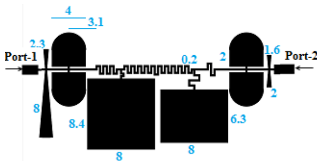
شکل ۹: طرح نهایی فیلتر پایین‌گذر پیشنهادی
