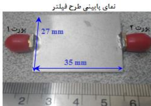
شکل ۱۰: نمونه ساخته شده فیلتر پایین‌گذر پیشنهادی
