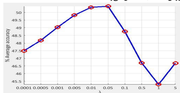
شکل ۹: ارزیابی دقت روش EDA برای مقادیر مختلف پارامتر \lambda (نمایش بهتر به صورت رنگی)
