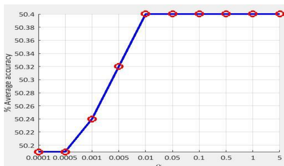
شکل ۶: ارزیابی دقت روش EDA برای مقادیر مختلف پارامتر \alpha (نمایش بهتر به صورت رنگی)
