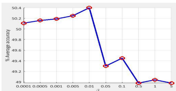
شکل ۷: ارزیابی دقت روش EDA برای مقادیر مختلف پارامتر \beta (نمایش بهتر به صورت رنگی)
