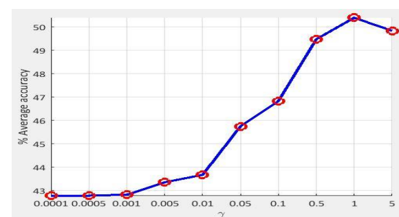
شکل ۸: ارزیابی دقت روش EDA برای مقادیر مختلف پارامتر \gamma (نمایش بهتر به صورت رنگی)
