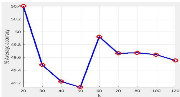
شکل ۵: ارزیابی دقت روش EDA برای مقادیر مختلف پارامتر k (نمایش بهتر به صورت رنگی)
