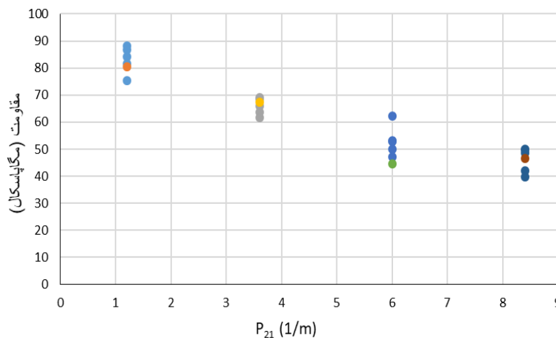
شکل ۷: مقاومت توده سنگی مدلسازی شده
