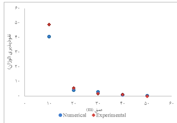
شکل ۱۰: مقایسه نفوذپذیری بدست آمده از تحلیل عددی (برده آب‌بند به عمق ۴۰m و زاویه ۱۷ درجه) و نتایج آزمایشگاهی
