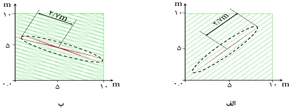
شکل ۵: مدل‌سازی عددی تزریق و برآورد شعاع نفوذ دوغاب در تکیه‌گاه‌های راست (الف) و چپ (ب) سد سردشت
