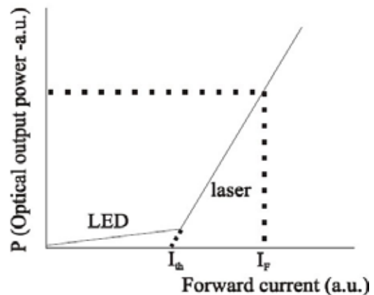
شکل ۳: مقایسه توان نوری خروجی ال‌ای‌دی و لیزر
