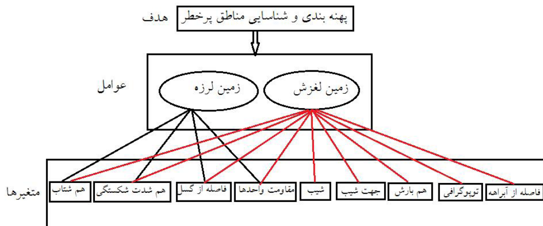
شکل ۲. نحوه ارتباط بین فاکتورهای موثر در وقوع زمین لرزه و زمین لغزش و ارتباط شبکه‌ای آنها (مقایسات زوجی هم بین متغیرها و هم بین عوامل صورت می گیرد. به عبارتی در اینجا ما سه بار مقایسه زوجی انجام می دهیم.
