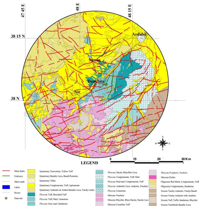
شکل ۳: نقشه زمین‌شناسی منطقه مورد مطالعه (نقشه‌های زمین‌شناسی ۱/۱۰۰۰۰۰ سازمان زمین‌شناسی با اصلاحات عمده حاصل از پیمایش‌های صحرایی).
