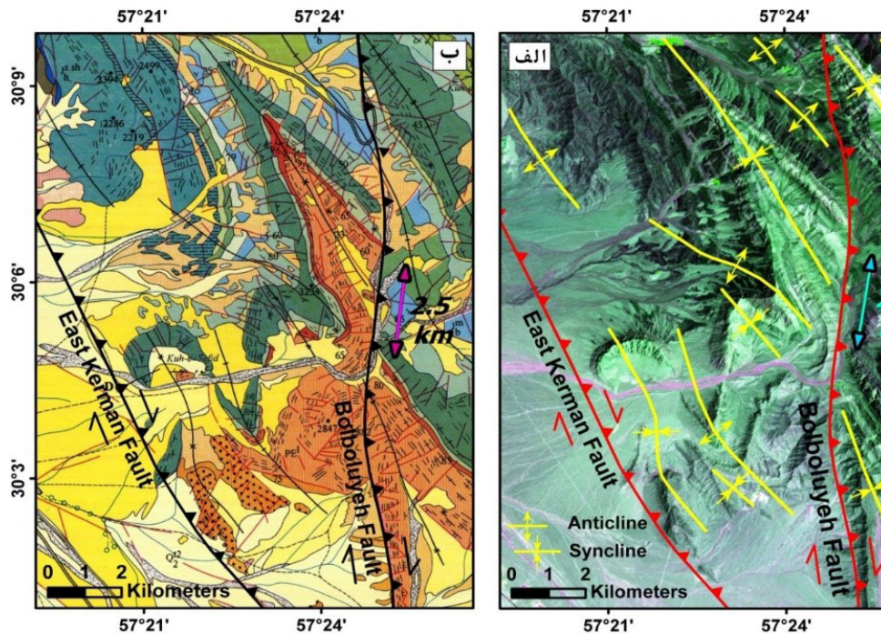
شکل ۲۱: الف) تصویر آستر از جابه‌جایی ۲/۵ کیلومتری یال خاوری ناودیس به همراه چین خوردگی‌های موجود داخل گوه ساختاری گسل بلبلویه و گسل خاور کرمان. ب) نقشه زمین‌شناسی تصویر الف (بر گرفته از نقشه ۱/۱۰۰۰۰ کرمان - عزیزان و همکاران (۱۳۷۸)).
