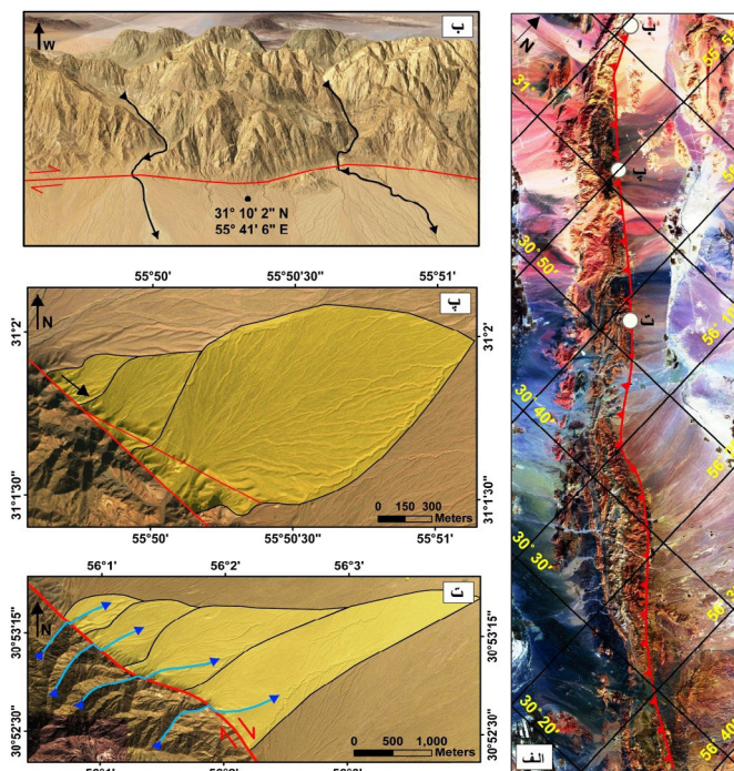
شکل ۱۸: الف) موقعیت گسل جرفاک در شمال خاور رشته کوه داوران. ب) جابه‌جایی ۱۵۰ متری راستگرد آبراه‌ها در قسمت شمال باختر گسل. ب) برش در مخروط افکنه‌ها (پ) کج‌شدگی مخروط افکنه‌ها. ت) جابه‌جایی آبراه‌ها در امتداد گسل.
