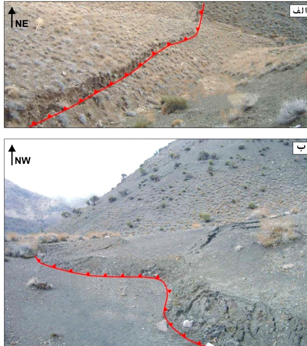
شکل ۱۳: گسیختگی حاصل از زمین‌لرزه ۱۳۸۳ داهوئیه زرنده. الف) بخش خاوری گسل داهوئیه. ب) بخش باختری گسل داهوئیه (عکس‌ها برگرفته از گروه لرزه زمین‌ساخت سازمان زمین‌شناسی و اکتشافات معدنی کشور است).
