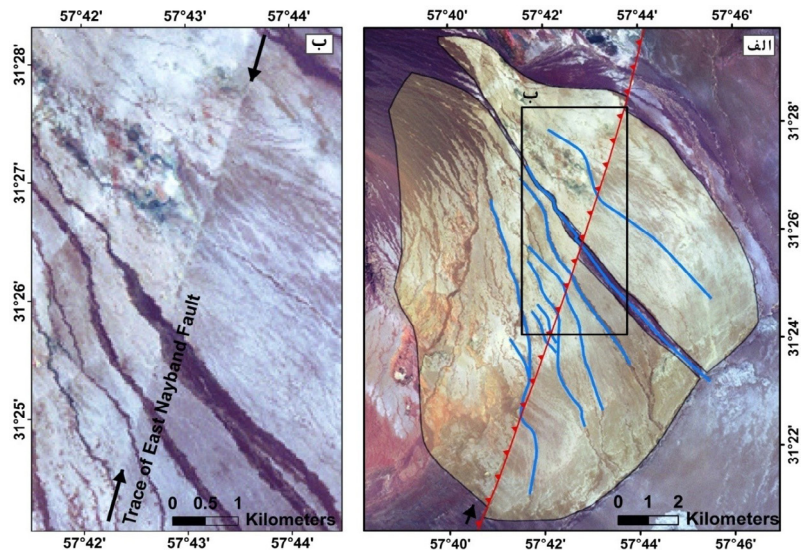
شکل ۴: الف) جابه‌جایی راستگرد ۵۰۰ متری مخروط افکنه و آبراهه‌ها در امتداد گسل خاور نایبند. ب) اثر گسل خاور نایبند و جابه‌جایی آبراهه‌ها از نمای نزدیک‌تر (Rashidi et al., 2018).
