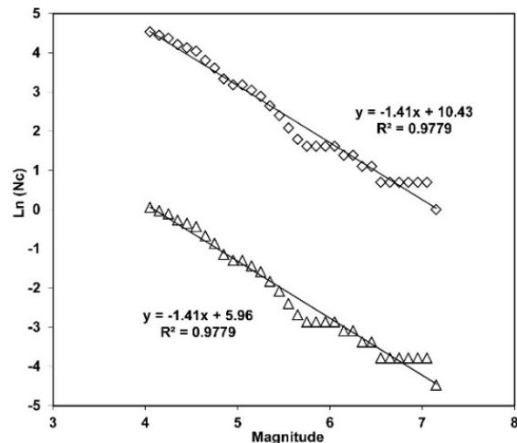
شکل ۲. ضرایب لرزه‌خیزی در گستره ۱۵۰ کیلومتری جنوب تهران
