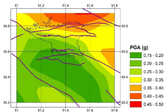
شکل ۸. بیشینه شتاب افقی ساختگاه سنگی بدون در نظر گرفتن گسل‌های جنوب تهران
