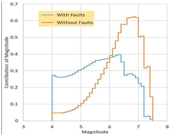
شکل ۱۳. سهم بزرگ‌های مختلف در ایجاد خطر لرزه‌ای دوره بازگشت ۴۷۵ سال
