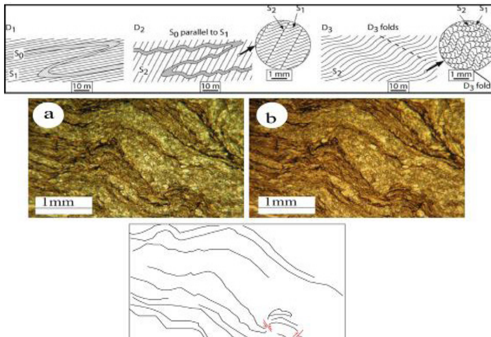
شکل ۲۹- تصویر میکروسکوپی از فیلیت دانه درشت منطقه قشلاق، برگ‌وارگی کنگره‌ای از نوع S_2 (شمال غرب - جنوب شرق) و در بال سمت راست دارای ریز گسل می‌باشد. برش موازی خط‌وارگی (XY plane) و عمود بر برگ‌وارگی (XZ plane) است، (a) نور پلاریزه (b) نور ساده.
