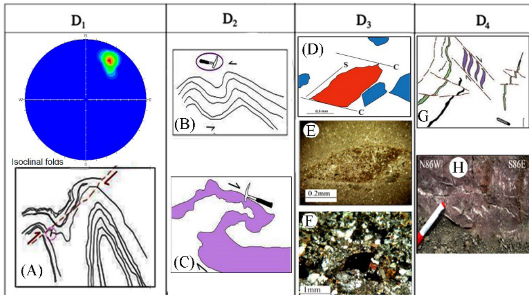
شکل ۳۴- خلاصه‌ای از ساختارهای اندازه‌گیری شده (تصاویر استریوگرافیک) و مشاهده شده در صحرا، A- فاز دگرشکلی D1، ساختارهای ایجاد شده در این فاز دگرشکلی، چین‌های هم‌شیب، B, C- فاز دگرشکلی D2، ساختارهای رخ داده در این فاز دگرشکلی، B: چین‌های برشی از نوع S شکل و C: چین‌های برشی از نوع Z شکل، D, E, F- فاز دگرشکلی D3، از ساختارهای ایجاد شده در این مرحله دگرشکلی، می‌توان ساختار S-C و بلورهای ماهی‌گون نام برد. D: ساختار S-C، E, F: بلورهای ماهی‌گون، G, H- فاز دگرشکلی D4، ساختارهای رخ داده در این فاز دگرشکلی، G, H: رگه‌های پوششی.
