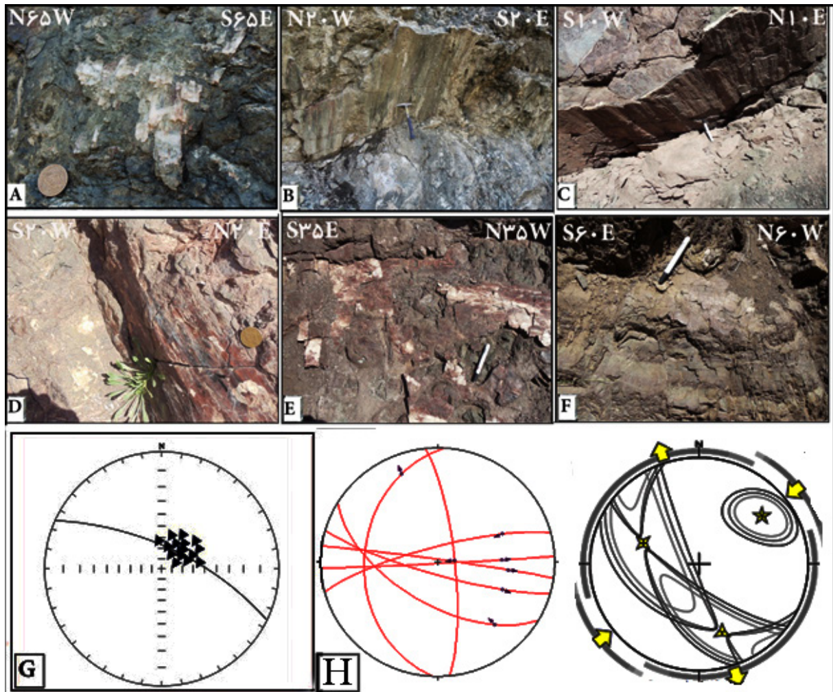
شکل ۱۶- A: خطواره سایشی کلسیت رشته‌ای در شیست‌های سبز میلونیتی شده در قچی گران حصار. جهت حرکت در عکس به طرف بالا می‌باشد. B: شیار خوردگی‌های روی صفحه گسل در شیست‌های میلونیتی در نزدیک روستای حصار جهت حرکت در عکس به طرف بالا می‌باشد. C: شیار خوردگی روی صفحه گسل در شیست‌های میلونیتی جاده حصار جهت حرکت به طرف بالا می‌باشد. D: شیار خوردگی روی صفحه گسل در آهک‌ها جاده حصار، جهت حرکت به طرف بالا می‌باشد. E: خطواره سایشی کوارتز رشته‌ای در شیست‌های سبز میلونیتی شده در نزدیکی روستای حصار، جهت حرکت در عکس به طرف راست می‌باشد. F: خطواره سایشی کلسیت رشته‌ای در شیست‌های سبز در نزدیکی روستای حصار، جهت حرکت به طرف چپ می‌باشد. G: خطواره‌های لغزشی بر روی صفحه گسل حصار-کوجوک. H: نتایج تحلیل انجام شده برای به دست آوردن متوسط رژیم تنش در منطقه قریس.
