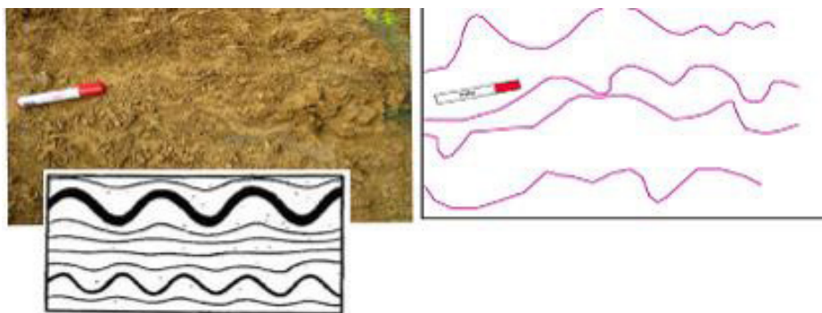
شکل ۱۸- چین‌خوردگی ناهماهنگ در کالک شیبست‌های روستای قریس، جهت دید عکس ۲۹۰°N
