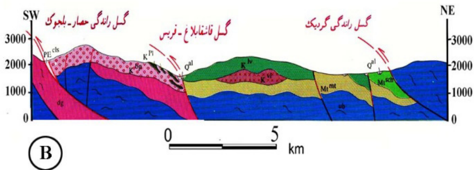
شکل ۶- A- نقشه‌ی گسل‌های منطقه مورد مطالعه با تغییرات کلی (اقتباس از رادفر و امینی، ۱۳۷۸، مطالعات صحرائی)، B- مقطع عرضی از گسل‌های منطقه در جهت شمال شرق - جنوب غرب.
