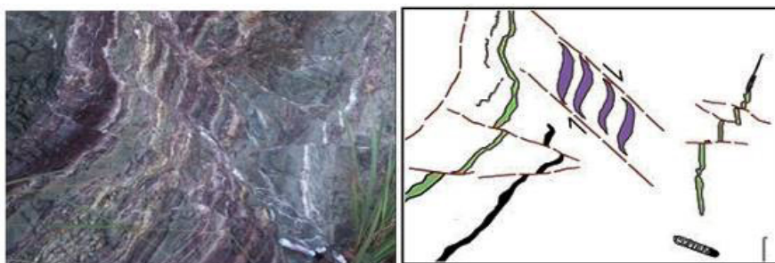
شکل ۲۸- نمایی از رگه‌های پوششی گرد در منطقه حصار، جهت دید عکس N345^\circ
