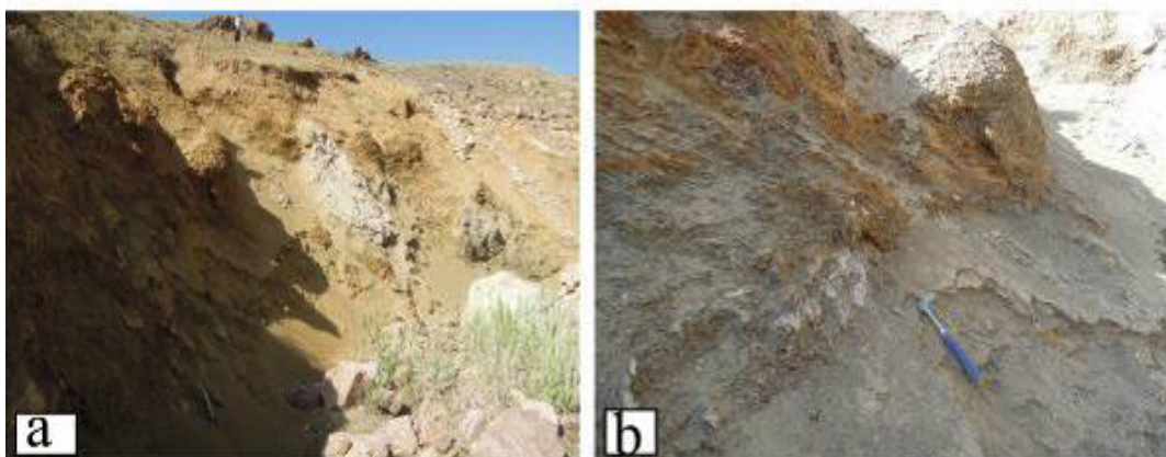
شکل ۱۳- (a,b) نمایی نزدیک از گوز گسل ناشی از گسل معکوس قریس - قشقابلاغ در منطقه گوگردلیق جهت دید شمالی - جنوبی.
