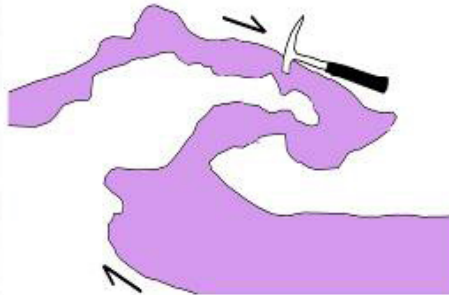
شکل ۲۱- چین خوردگی برشی از نوع Z شکل بر رگه‌های چرت در مسیر روستای حصار، جهت دید عکس N325^{\circ} می‌باشد.
