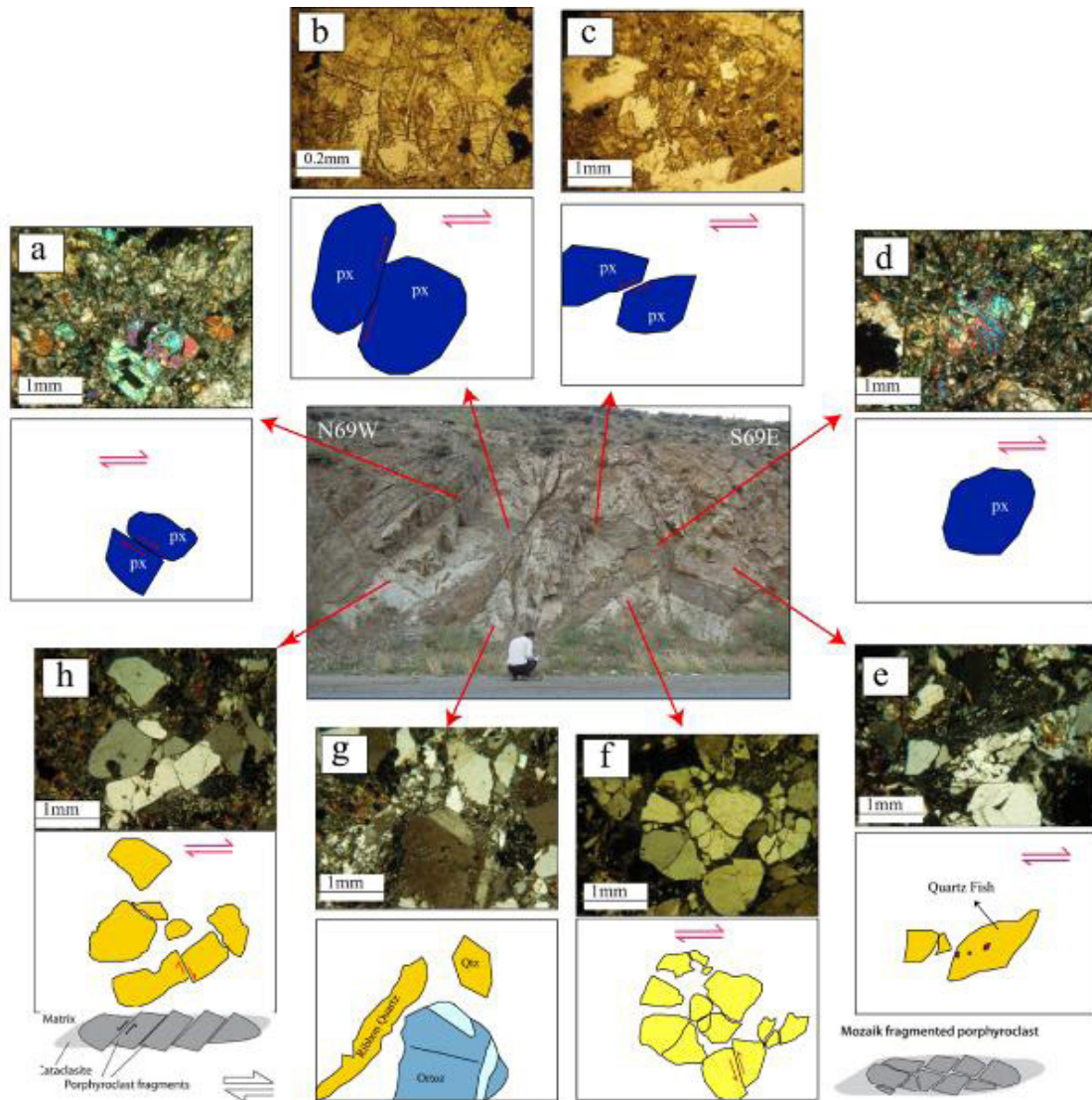
شکل ۱۷- ریز ساختارهای مطالعه شده در دایک پریدوتیتی و توده ریولیتی (بالای راه‌دارخانه گوردیک، جنوب شرقی منطقه قریس) شکل‌های a, b, c, d از دایک پریدوتیتی و شکل‌های e, f, g, h از توده ریولیتی می‌باشد. شکل a, b, c, پیروکسن قفسه‌کتابی، شکل d پیروکسن ماهی جهت حرکت راست گرد می‌باشد. شکل e بلور کوارتز ماهی شکل با ادخال‌های اپیدوتیتی جهت حرکت راست گرد می‌باشد. شکل f پورفیر و کلاست برش خورده و کاتاکلاستی بلورهای کوارتز و برش‌گسلی می‌باشد. شکل g پورفیر و کلاست و تأثیر ریز گسل بر روی آن را نشان می‌دهد. شکل h بلور قفسه‌کتابی کوارتز را نشان می‌دهد. در شکل‌های f, h سیالات کلریتی در شکستگی‌های بلورهای کوارتز وجود دارد. b, c ساده نور پلاریزه. در تمامی عکس‌ها سوی برش راست گرد، برش موازی خط‌وارگی (XY plane) و عمود بر برگ‌وارگی (XZ plane) است.
