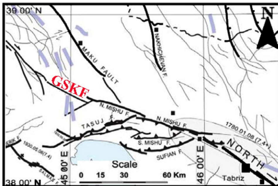
شکل ۷- تقسیم‌بندی گسل‌های فعال منطقه شمال تبریز - خوی و گسل افشانه‌ای گیلاتو-سیه چشمه-خوی (GSKF) (اقتباس از Kara-khanian et al., 2004).
