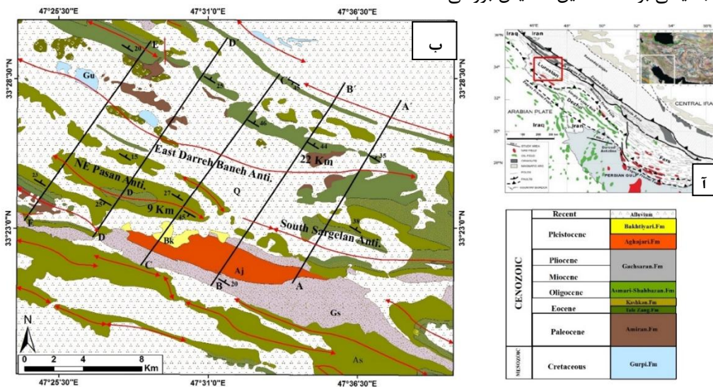
شکل ۱. (ا) نقشه ساختاری منطقه زاگرس و حوضه پیش‌بوم همراه با ورقه عربی که موقعیت منطقه بررسی شده با چهار گوش قرمز مشخص شده است [۵۸]. (ب) نقشه زمین‌شناسی منطقه بررسی شده [۳۲]-[۵۵] که بیش‌تر رخنمون‌های سطحی را سازندهای آسماری و جوان‌تر پوشانده‌اند.
