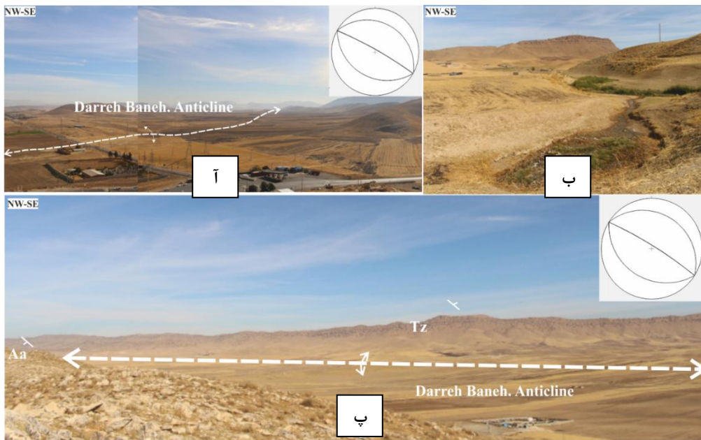
شکل ۷. آ) هسته تاقدیس دره‌بانه در امتداد نیمرخ BB' ، ب) تشکیل چشمه‌های نفتی و گازی در نزدیکی یال شمالی تاقدیس دره‌بانه، پ) محور تاقدیس دره‌بانه با رخنمونی از سازندهای آسماری و تله‌زنگ در بال‌ها As و Tz به ترتیب تله‌زنگ و آسماری را نشان می‌دهند.
