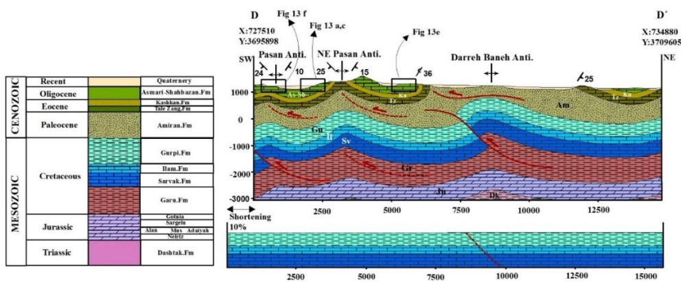
شکل ۱۲. مقطع ساختاری DD' عمود بر محور تاقدیس‌های پاسان، پاسان شمال شرق و دره‌بانه ترسیم شده است. رانندگی‌های سطحی و عمقی با ریشه در سطوح جدایشی تاقدیس دره‌بانه شده است.
