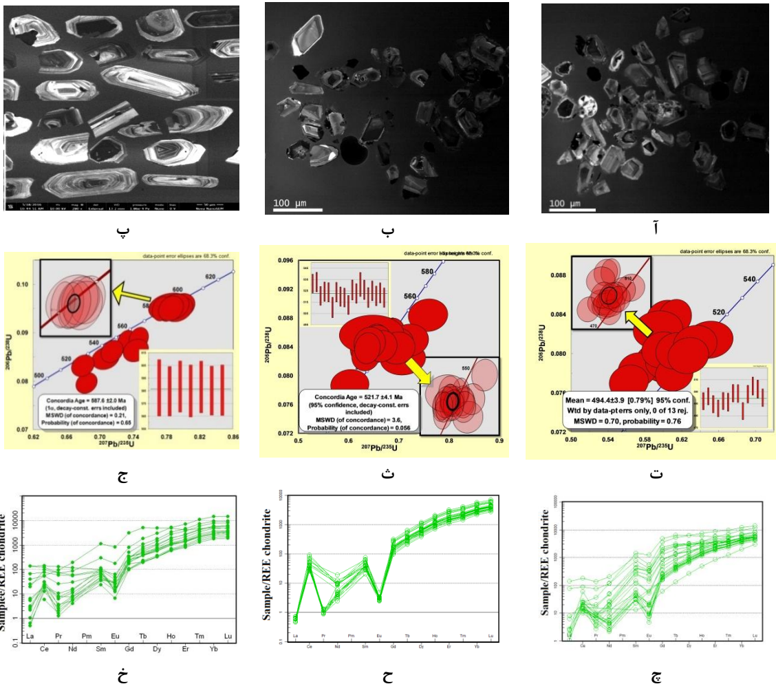
شکل ۸. الف، ب و پ) تصاویر کاتادلومینسانس از زیرکن‌های استخراج شده از متاریولیت‌های ماجراد و شترکوه. ت، ث و ج) نمودارهای سازگاری مبتنی بر نتایج سن‌سنجی به روش U-Pb. چ، ح، خ) نمودارهای تغییرات عناصر خاکی-نادر به‌هنگار شده نسبت به کندریت بونتون [۳۹] برای زیرکن‌های استخراج شده از نمونه‌های متاریولیتی ماجراد.
