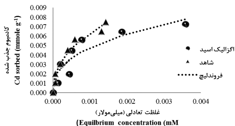
شکل ۶- همدمای جذب کادمیوم توسط بخش رس خاک برآزش یافته با مدل فروندلیچ.
