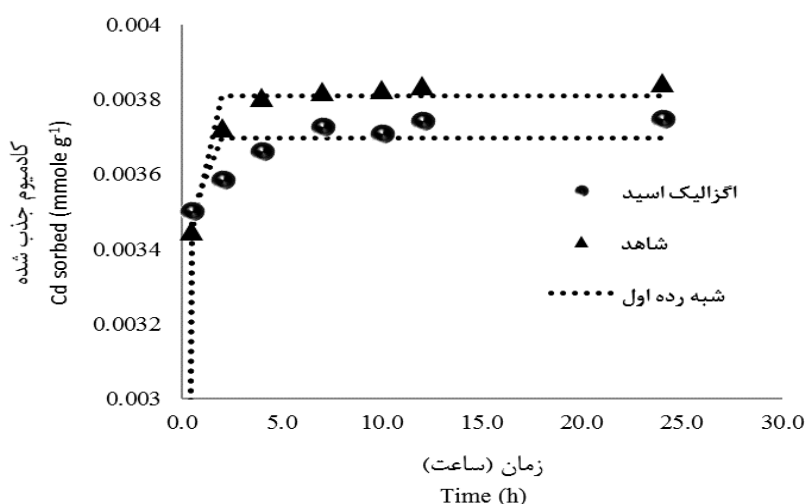
شکل ۳- برازش مدل شبه‌مرتبه اول بر جذب وابسته به زمان کادمیوم توسط بخش رس خاک.
