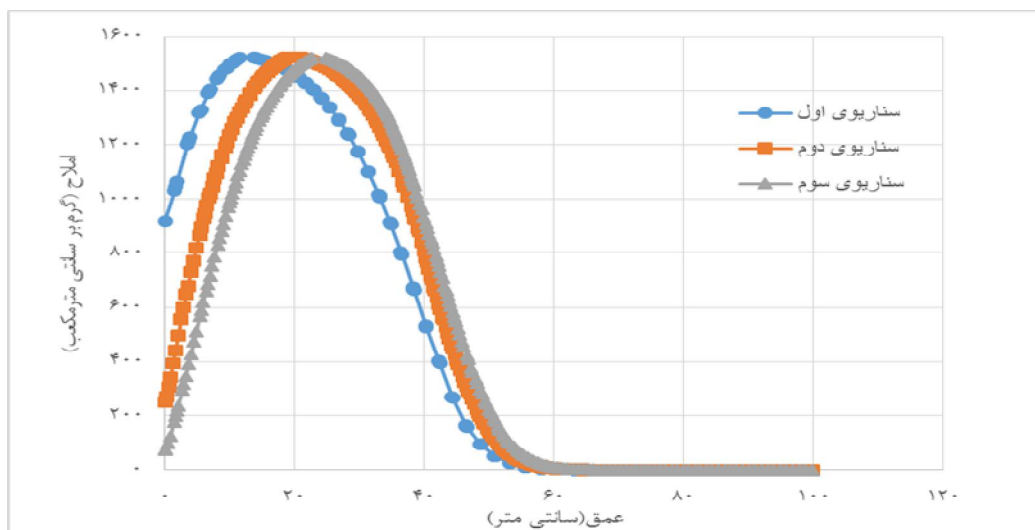
شکل 4- مقایسه تغییرات املاح نسبت به عمق در سناریوهای تعریف شده
