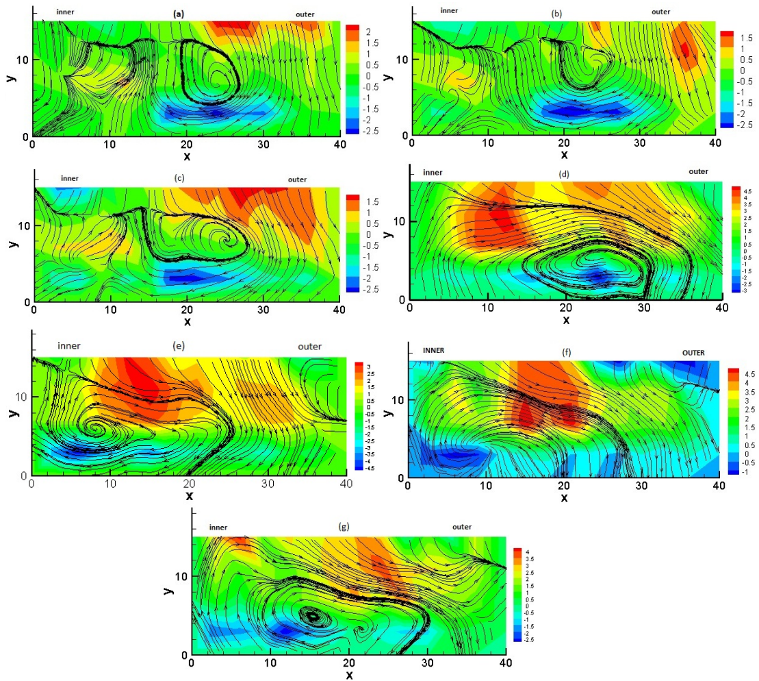
شکل ۱۰- خطوط جریان عرضی و توزیع سرعت در مقاطع عرضی برای دبی ۱۵ لیتر بر ثانیه و زبری ۰/۵ میلی متر a: ۳۰ سانتی متر بالادست قوس b: مقطع صفر درجه c: مقطع ۲۰ درجه d: مقطع ۴۰ درجه e: مقطع ۷۰ درجه f: مقطع ۹۰ درجه g: ۳۰ سانتی متر پایین دست قوس
