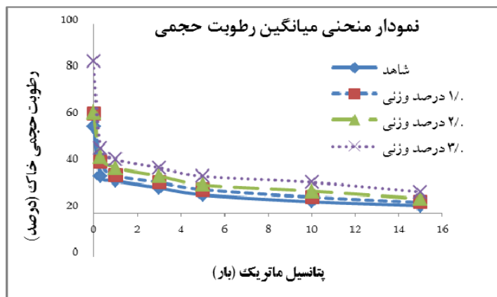
شکل ۲- منحنی میانگین رطوبت حجمی خاک در اثر کاربرد سطوح مختلف پلیمر سوپر جاذب A300
