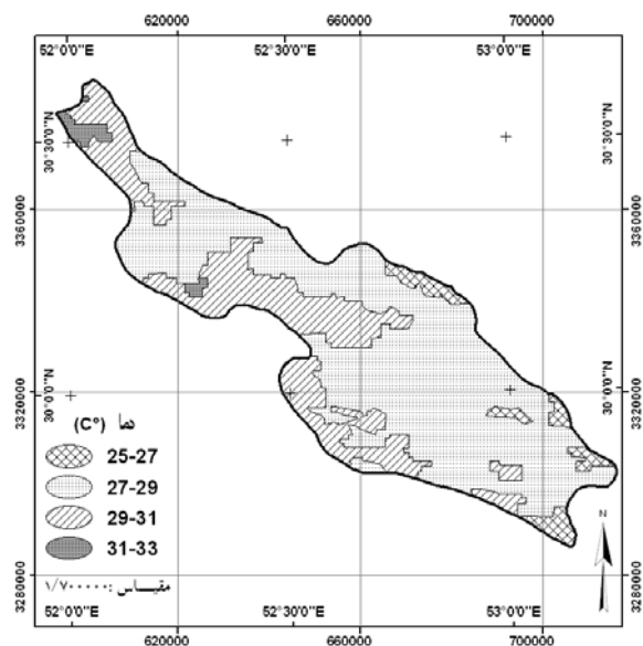
شکل ۳- دمای تاج پوشش محصول گندم در منطقه مرودشت در تاریخ ۱۳۸۸/۳/۵ ساعت ۱۱:۴۰ محلی
