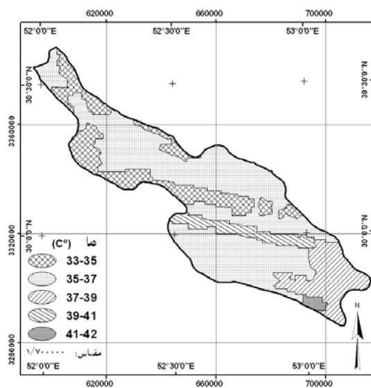
شکل ۴- دمای تاج پوشش محصول گندم در منطقه مرودشت در تاریخ ۱۳۸۸/۴/۲ ساعت ۱۲:۰۴ محلی
