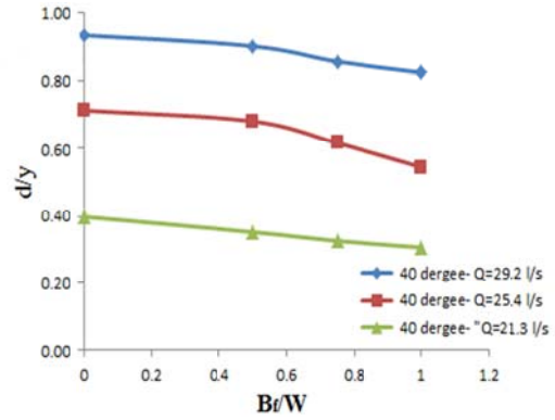
شکل ۱۳- تأثیر تغییر بال آبشکن بر آبشستگی در \phi=40^\circ
