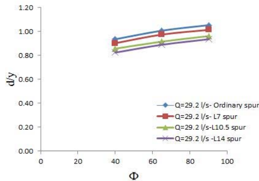
شکل ۸- تأثیر موقعیت آبشکن بر آبستنگی با Q=29/2 لیتر بر ثانیه
