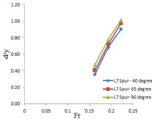
شکل ۹- تأثیر عدد فرود بر آبشستگی در آبشکن ساده / شکل ۱۰- تأثیر عدد فرود بر آبشستگی در B_f=7 سانتی متر
