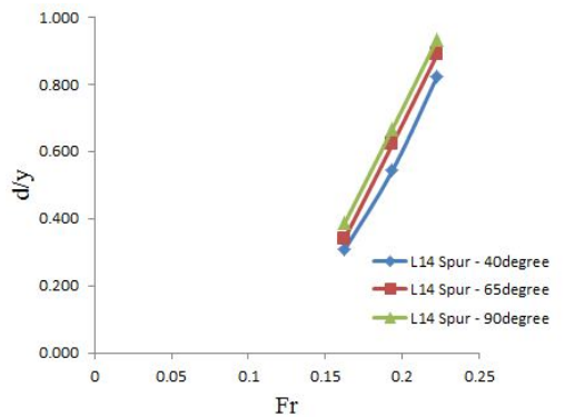
شکل ۱۱- تأثیر عدد فرود بر آبشستگی در B_f=10,5 سانتی متر / شکل ۱۲- تأثیر عدد فرود بر آبشستگی در B_f=14 سانتی متر
