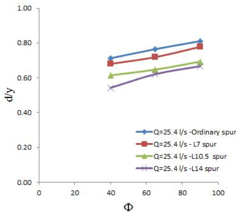
شکل ۷- تأثیر موقعیت آبشکن بر آبستنگی با Q=25/4 لیتر بر ثانیه
