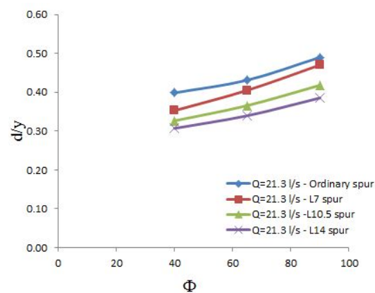
شکل ۶- تأثیر موقعیت آبشکن بر آبستنگی با Q=21/3 لیتر بر ثانیه
