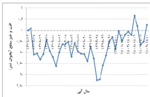
شکل ۶- الف) تراز آبخوان شبیه سازی شده دشت نیشاپور تحت سناریوی مدیریتی اول
