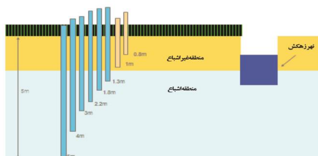
شکل ۵- نمایی شماتیک از کارگذاری لوله های پیزومتریک در یک نقطه از زمین
