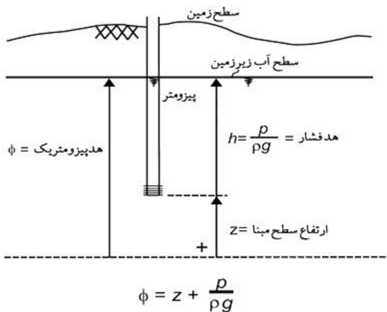
شکل ۲ - نمایش بار پیزومتریک
