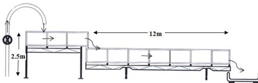
شکل ۱- شماتیکی از فلوم آزمایشگاهی مورد استفاده
