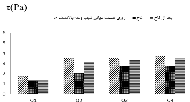
شکل ۷- مقادیر تنش برشی بستر در شیب ۰/۰۰۳
