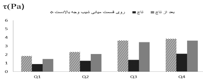
شکل ۶- مقادیر تنش برشی بستر در شیب ۰/۰۰۲
