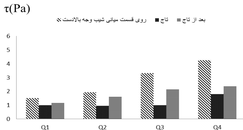
شکل ۵- مقادیر تنش برشی بستر در شیب ۰/۰۰۱
