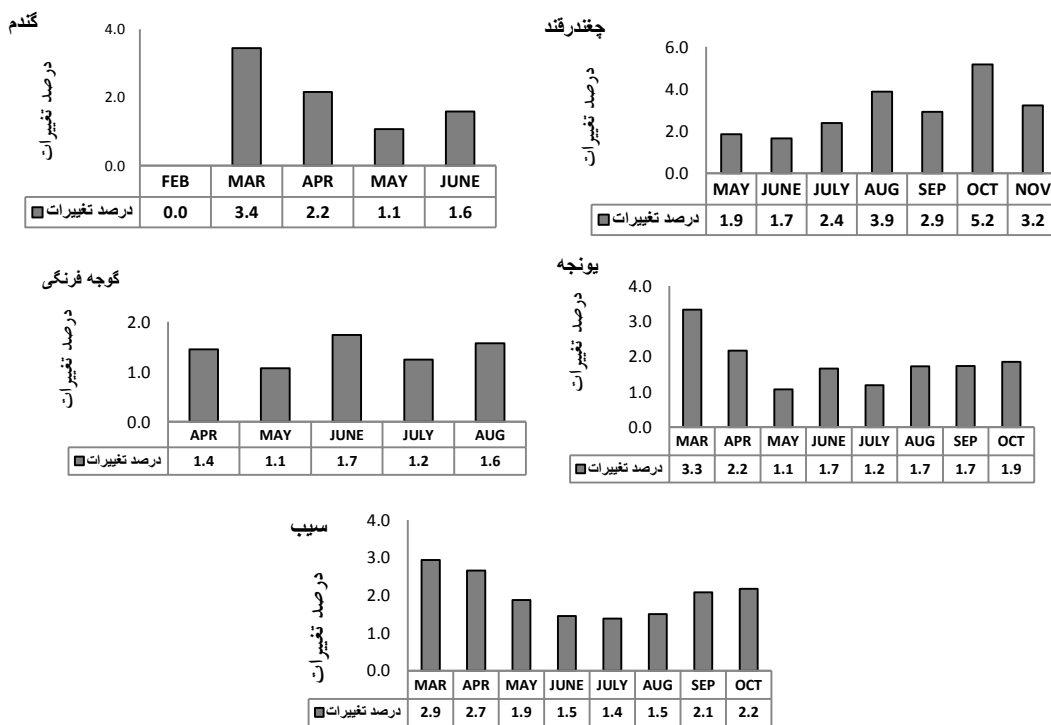
شکل ۱۰- درصد تغییرات نیاز آبی محصولات منتخب دشت مشهد در دوره ۲۰۰۹-۲۰۱۸ نسبت به دوره پایه در طول فصل رشد
