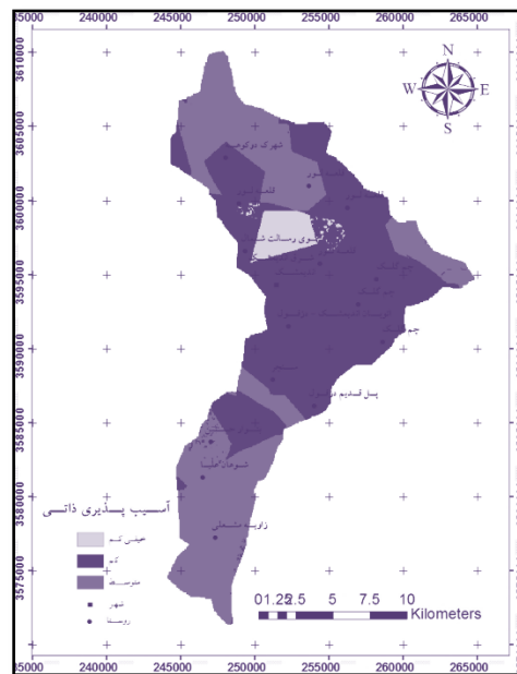
شکل (۴): نقشه آسیب‌پذیری ذاتی نهایی آبخوان اندیمشک شکل (۵): نقشه آسیب‌پذیری ویژه نهایی آبخوان اندیمشک
