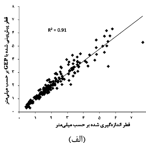
شکل (۸): مقایسه متوسط اندازه قطره‌های اندازه‌گیری شده از آزمایش‌ها با نتایج حاصل از مدل برنامه‌ریزی ژنتیک الف- داده‌های آموزش ب) داده‌های آزمون
