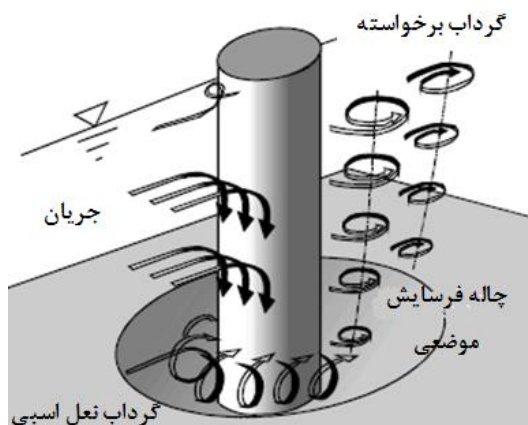
شکل (۱): شماتیکی از حفره آبشستگی و الگوی جریان اطراف پایه پل استوانه‌ای
