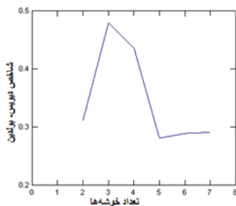
شکل (۳): مقادیر شاخص دیوبس-بولدین برای تعیین تعداد بهینه خوشه‌ها
