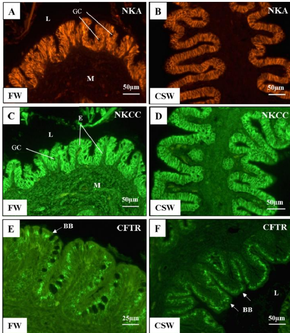
شکل ۲: مکان‌یابی پروتئین‌های ناقل یون NKA (A و B)، NKCC (C و D) و CFTR (E و F) به روش ایمونوهیستوشیمی در بافت دریچه مارپیچی روده بچه تاس‌ماهیان ایرانی ۳-۲ گرمی پس از ۱۰ روز نگهداری در آب شیرین (FW) و آب دریای خزر (CSW). BB: نوار مسواکی (Brush Border)؛ E: انتروسیت (Enterocyte)؛ GC: سلول‌های گبلیتی (Goblet Cells)؛ L: لومن (Lumen)؛ LP: لامبنا پروپیرا (Lamina Propira)؛ M: بافت ماهیچه‌ای (Muscle Tissue).
