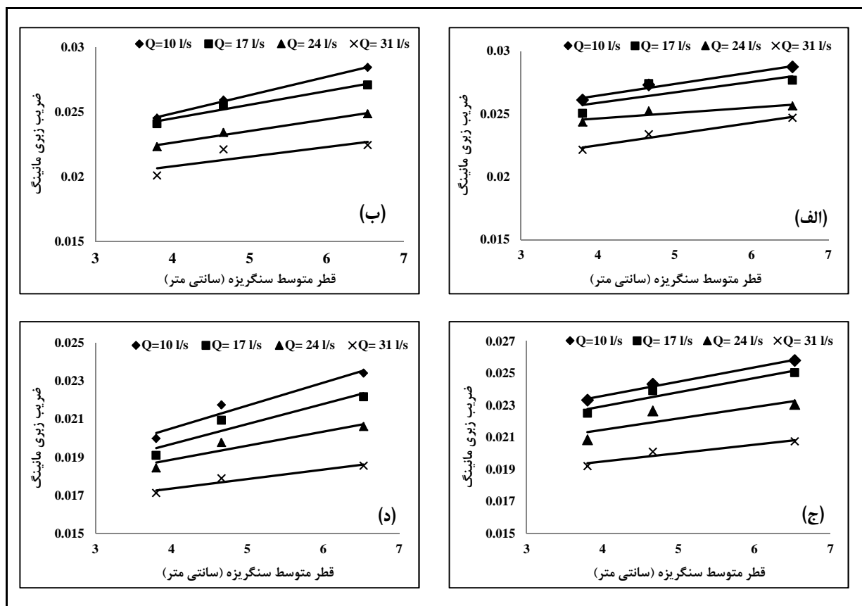
شکل ۶- تغییرات ضریب زبری مانینگ در برابر اندازه سنگریزه‌های شکسته تیز گوشه برای شیب‌های: (الف) ۱ درصد، (ب) ۱/۸ درصد، (ج) ۱/۶ درصد و (د) ۱/۴ درصد
