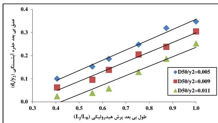
شکل ۸- تغییرات عمق بی‌بعد حفره آبستگي به‌ازاي طول بی‌بعد پرش هیدروليكي
