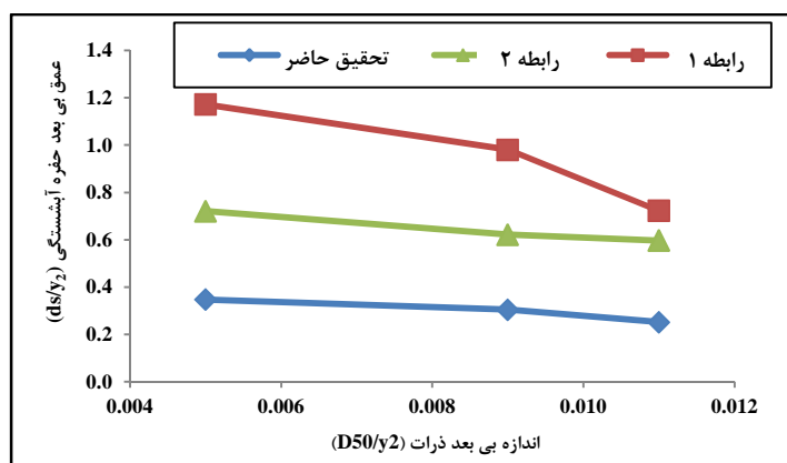
شکل ۹- تغییرات عمق بی‌بعد حفره آبستگي به‌ازاي اندازه بی‌بعد ذرات
