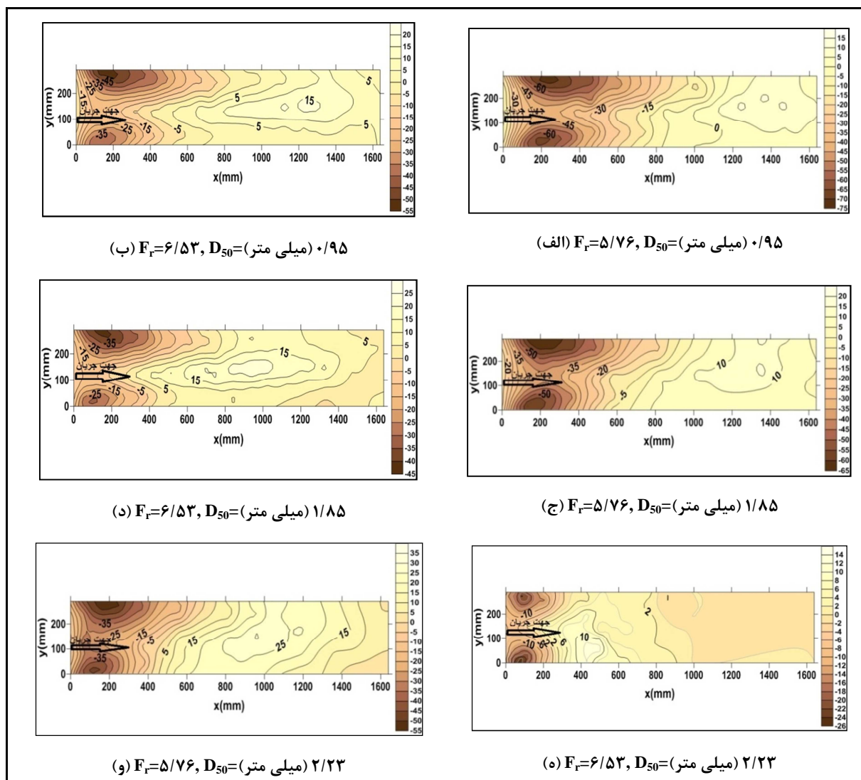
شکل ۶- پروفیل آبستنگی در پایین دست حوضچه آرامش پوشیده با المان های شش پایه
