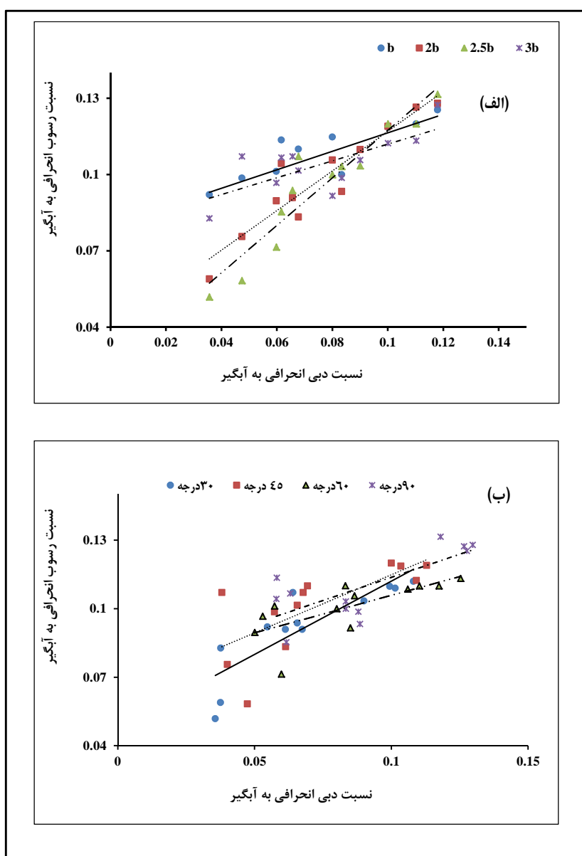
شکل ۵- نسبت رسوب انحرافی به آبگیر بر حسب نسبت دبی انحرافی
