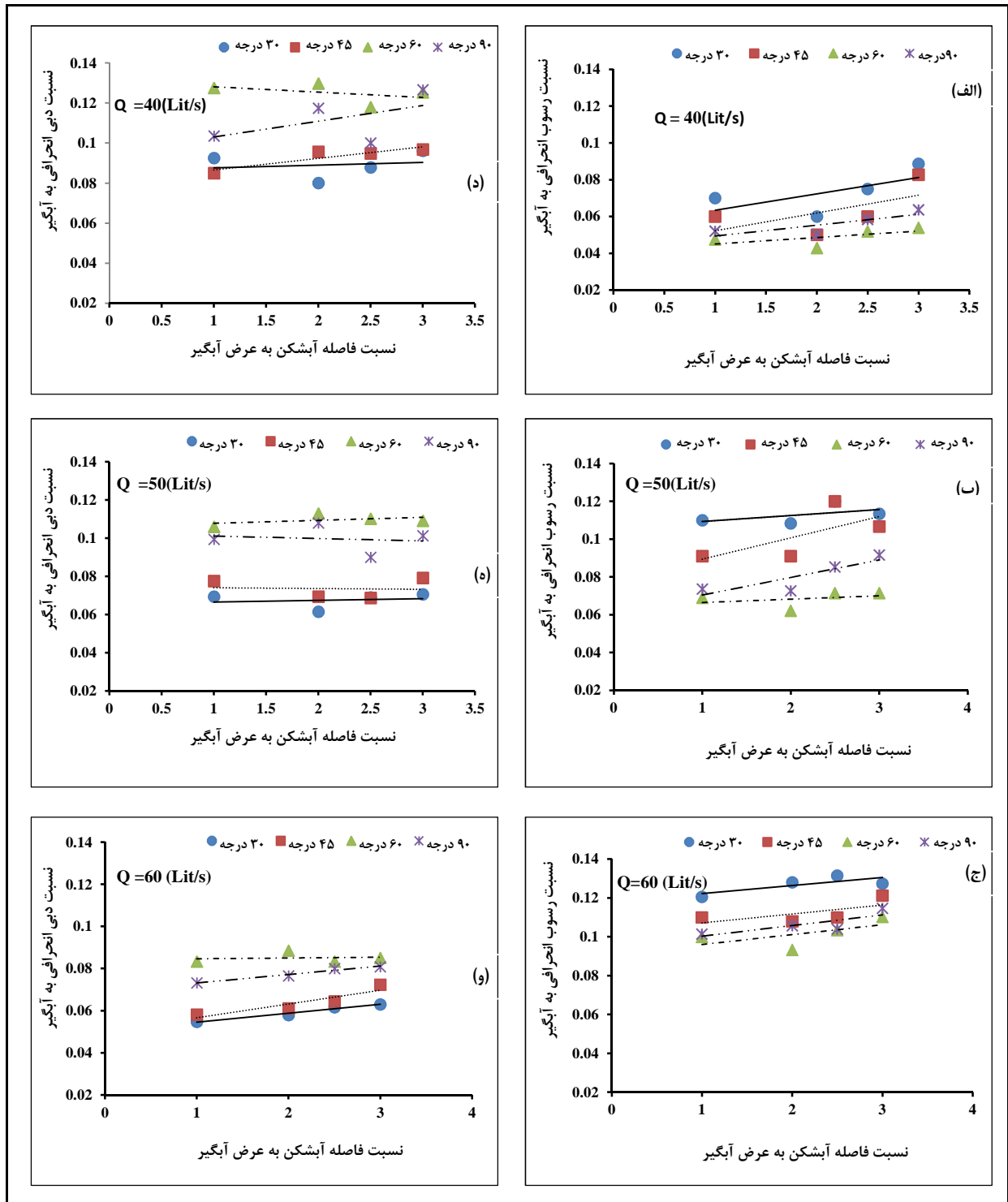
شکل ۶- رابطه بین پارامتر بدون بعد نسبت فاصله آبشکن به عرض آبیگر (L/b)
