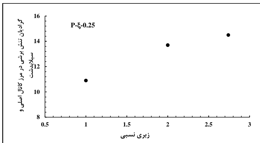
شکل ۱۶- مدلسازی عددی گرادینان تنش برشی مرزی در محل اتصال کانال اصلی و سیلابدشت به ازای زبری های مختلف
