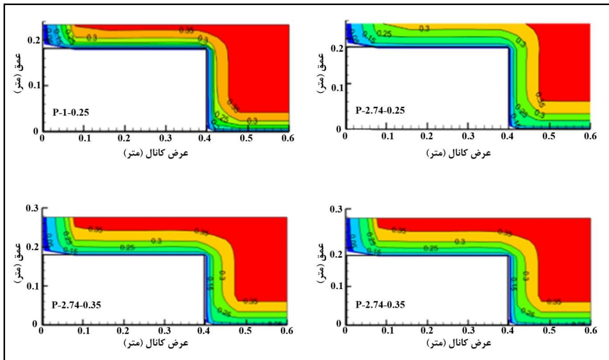
شکل ۱۰- نتایج مدل عددی توزیع سرعت جریان در کانال مرکب
