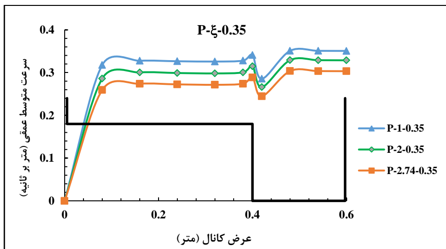
شکل ۱۲- مقایسه نتایج مدلسازی عددی سرعت متوسط عمقی جریان در عمق نسبی ۳۵٪ با زبری های مختلف
