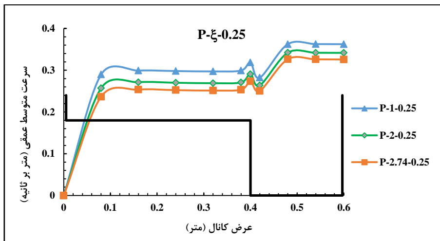
شکل ۱۳- مقایسه نتایج مدلسازی عددی سرعت متوسط عمقی جریان در عمق نسبی ۲۵٪ با زبری های مختلف اثر افزایش زبری بر تنش برشی مرزی
