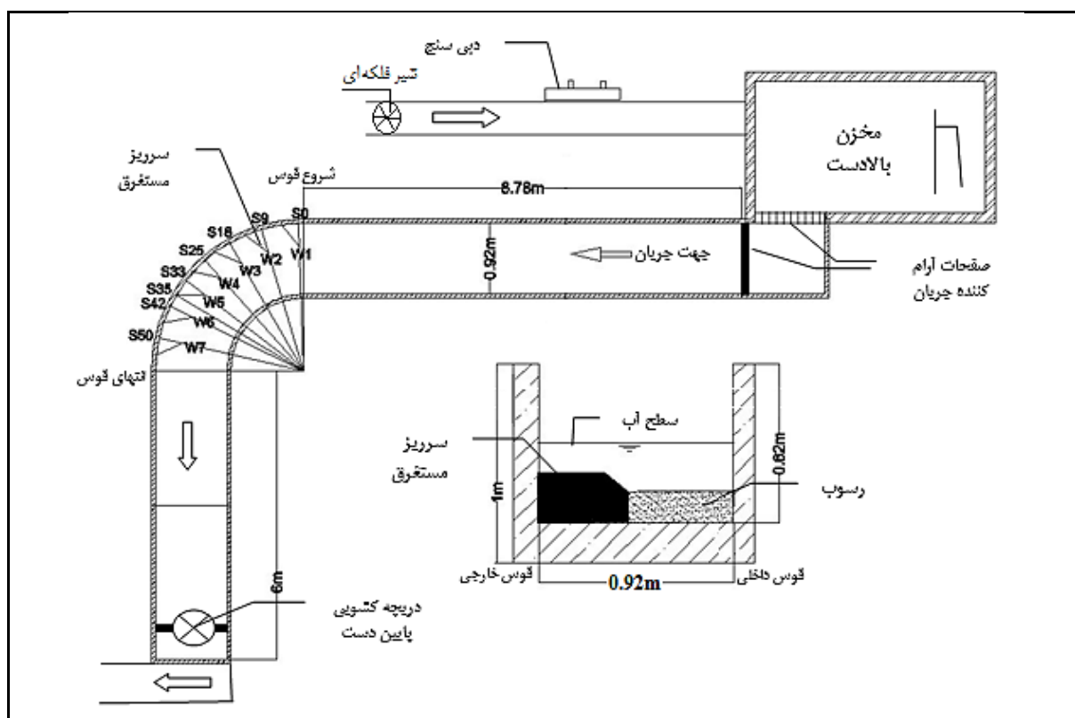
شکل ۱- تجهیزات آزمایشگاهی
