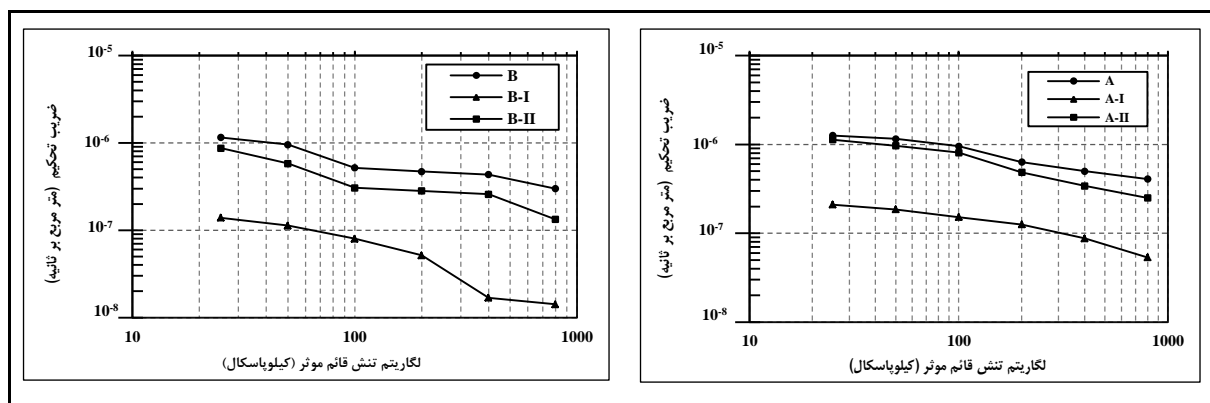
شکل ۶- نمودار ضرایب تحکیم روی نمونه‌های مورد آزمایش
