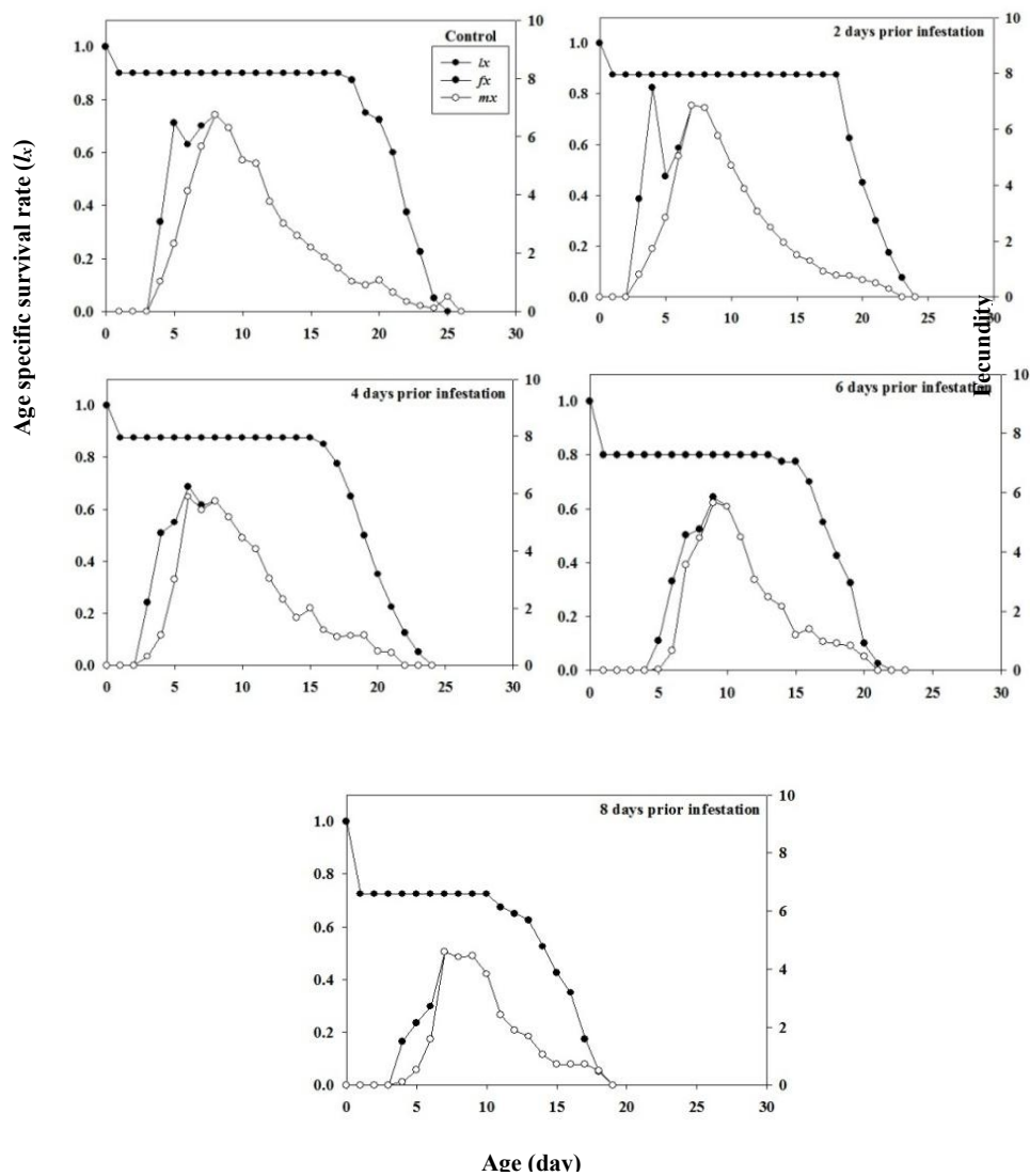
شکل ۳- منحنی‌های تغییرات باروری ویژه‌ی سنی - مرحله‌ای ( f_{xj} )، بقای ویژه‌ی سنی ( l_x ) و باروری ویژه‌ی سنی ( m_x ) شته جالیز روی تیمارهای مختلف پیش-آلودگی در رقم رویال.
