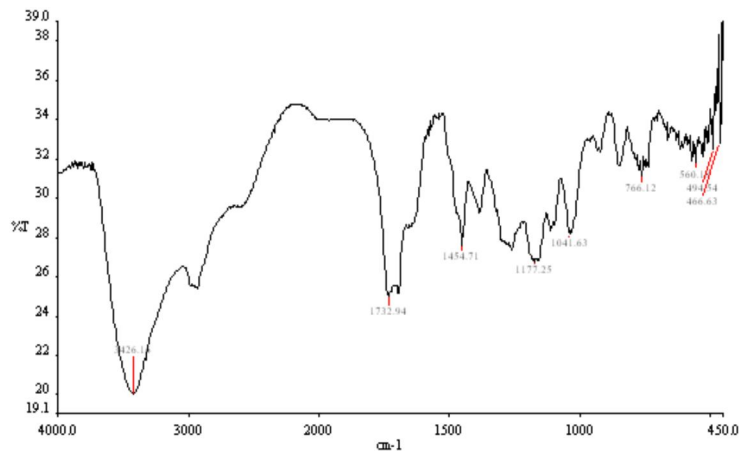
تصویر (۴): طیف FT-IR از فیبرهای داکسوریسین و PAMAM بعد از الکتروریسی
